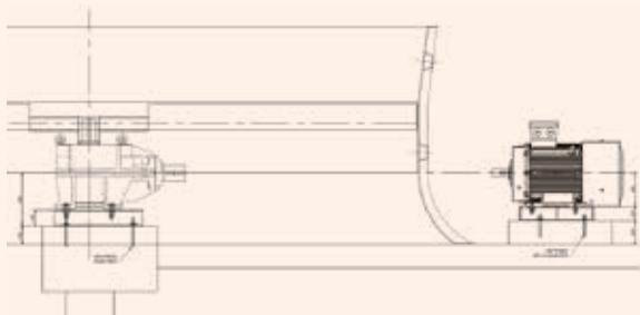
Tipico disegno in sezione del gruppo meccanico per l'installazione: allineamento del motore e del riduttore attraverso il ventilatore
